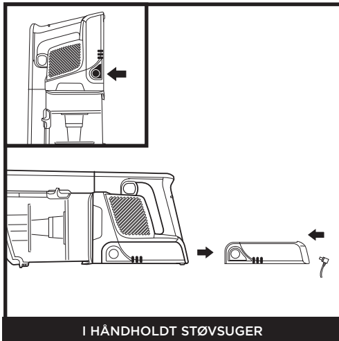
OPLADER TIL LITIUM-ION POWER PACK
